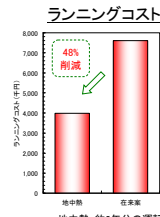
地中熱: 約5年分の運転実績値より。在来系: (融雪)電熱線方式 + (冷暖)空冷チラー + (暖房)灯油ボイラー
