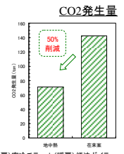
地中熱: 約5年分の運転実績値より。在来系: (融雪)電熱線方式 + (冷暖)空冷チラー + (暖房)灯油ボイラー
